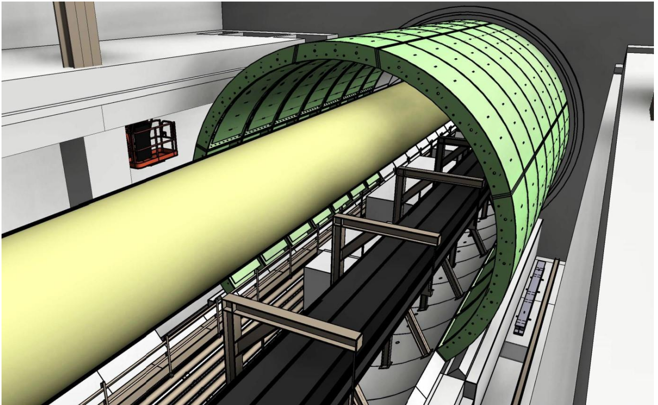
3D-Visualisierung des Tunnel-Modells zu Los 3 der Linie C der Metro in Toulouse (Bild: ©Implenia).
